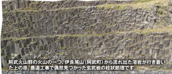
阿武火山群の火山の一つ、伊良尾山(阿武町)から流れ出した溶岩が行き着いた上の原。農道工事で偶然見つけた玄武岩の柱状節理です。
